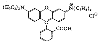
図 18. C. I. Basic Violet 10
