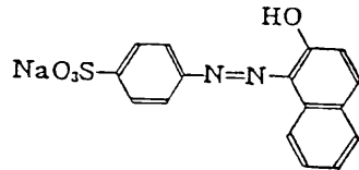
図 13. C.I. Acid Orange 7
