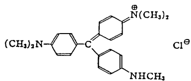
図 17. C. I. Basic Violet 1
