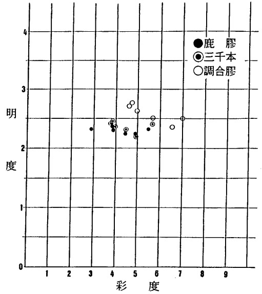
図3 杉板試料の明度・彩度の変化（薄い濃度）
