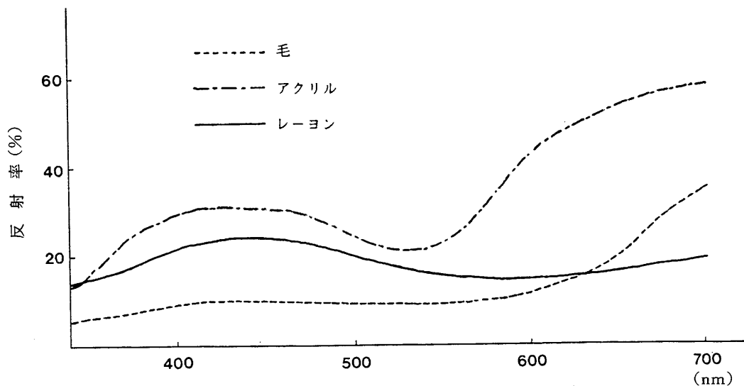
図4. Tulipanin による染布の反射率曲線
